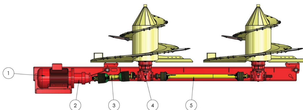
Figuur 9-1 Indirecte vijzelaandrijving
