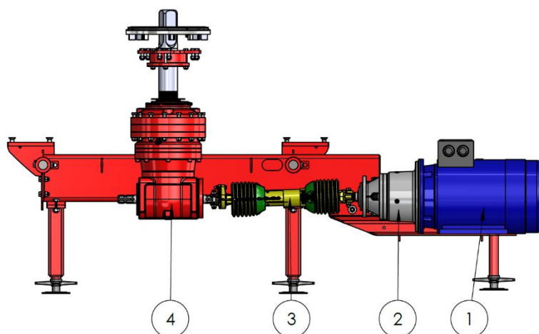
Figuur 9-2 Directe vijzelaandrijving
