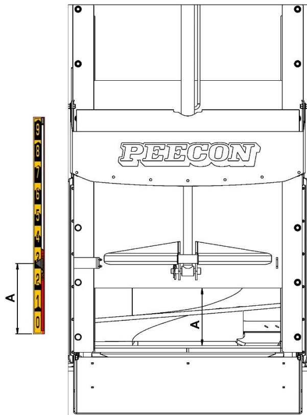
Figuur 9-7 Losdeur
