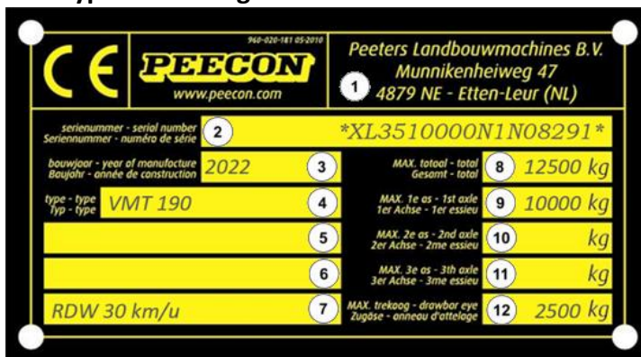
Figuur 2-1 Typeplaatje
